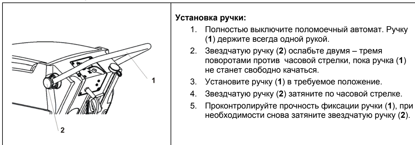
Рис. 8 Установка ручки
