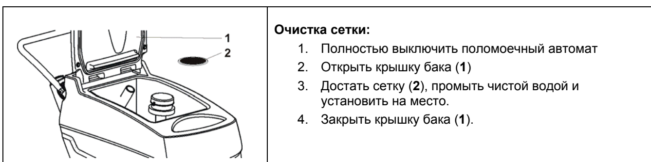
Рис. 17 очистка сетки
