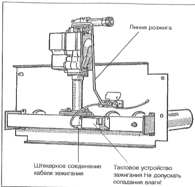
Рис. 33: Газовая горелка
