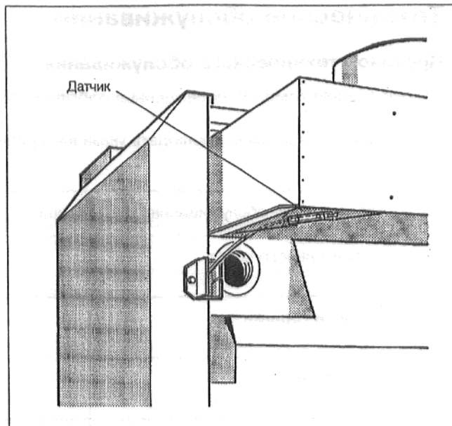
Рис. 26: Датчик устройства контроля отходящего газа
