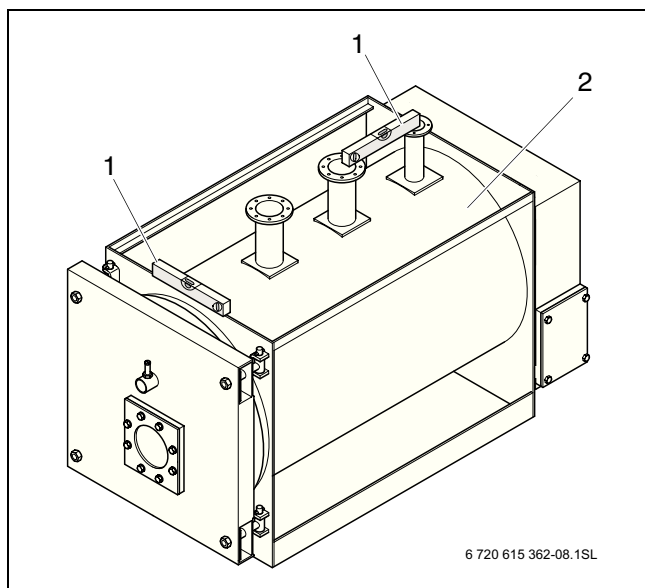
Рис 9 Выравнивание котла
