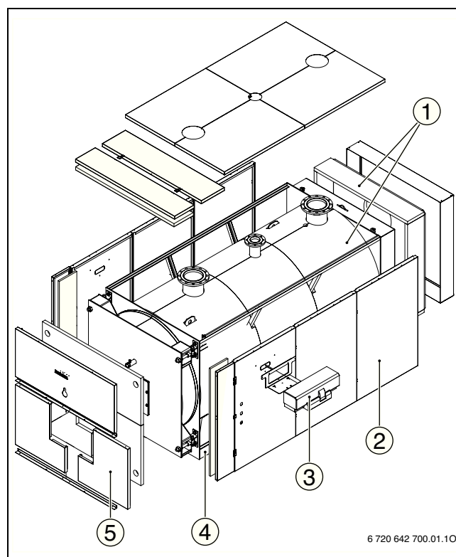
Рис 2 Специальный отопительный котёл Logano 1400-1850 кВт
