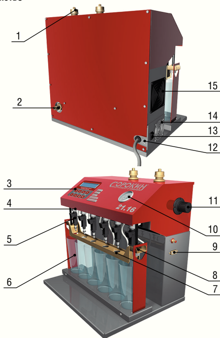
Рисунок 1 - Общий вид
