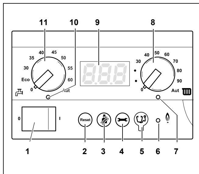
Рис. 5 Главный регулятор BC10
