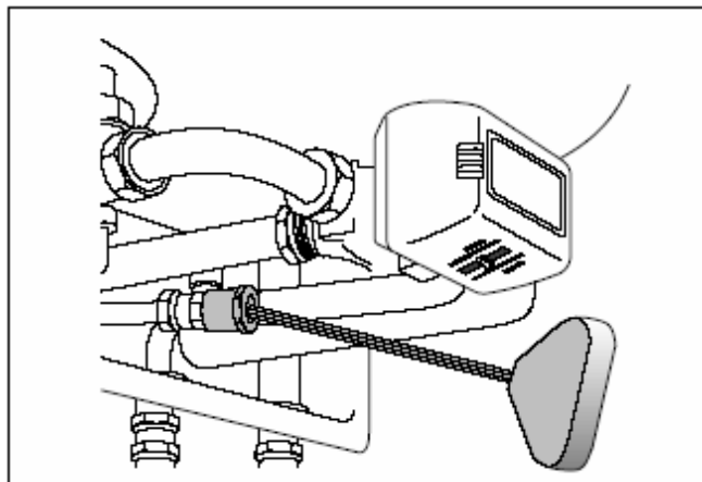
Рис. 23 Ограничитель расхода горячего водоснабжения
