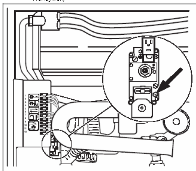
Рис. 20 Продувка газопровода подачи газа (арматура SIT)
