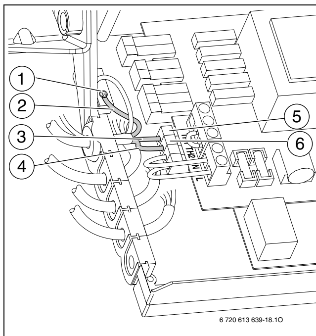
Рис 16 Подключение сетевого кабеля 230 В перем. тока
