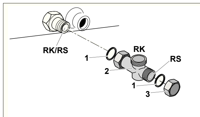
Рис. 17 Монтаж соединительного элемента обратной линии
