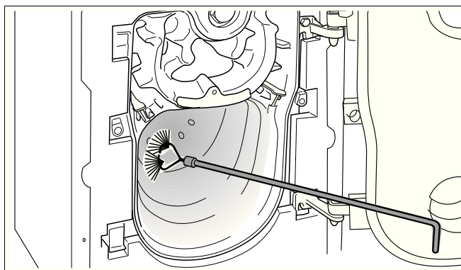
Рис. 42 Чистка топочной камеры
