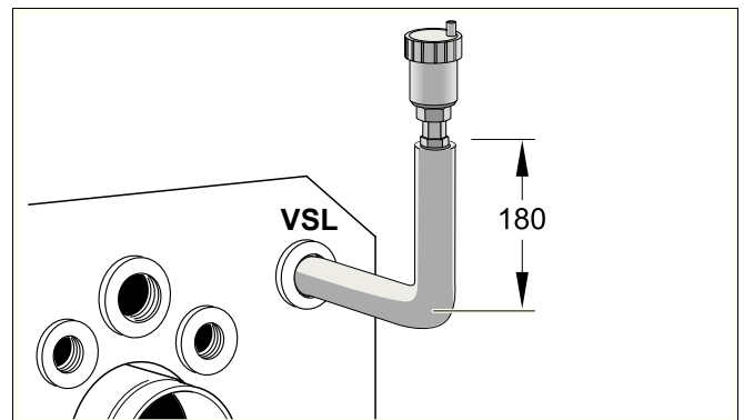
Рис. 20 Подключение воздушного клапана к предохранительной линии (размеры в мм)
