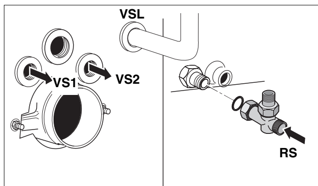
Рис. 22 Подключение бака-водонагревателя
