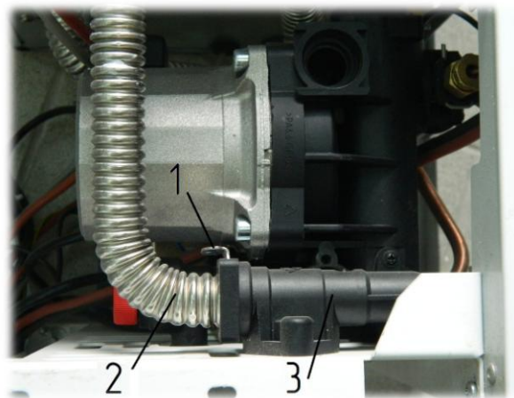
Рис. 18 Демонтаж клапана байпаса
