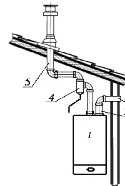
Рис. 4. Монтаж раздельного дымохода
