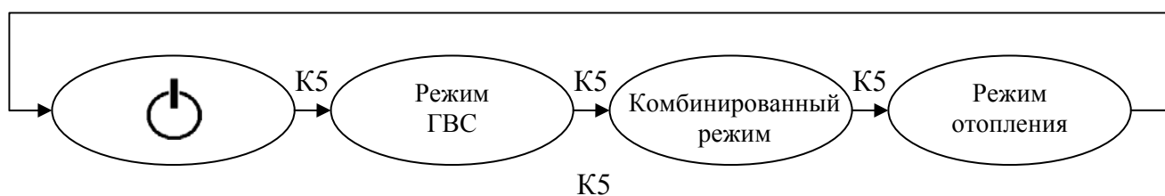
Рис. 5. Последовательность смены режимов работы котла
