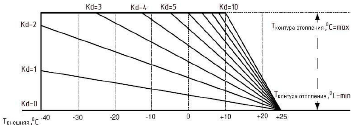
Рис. 6. График зависимости температуры в контуре отопления от внешней температуры
