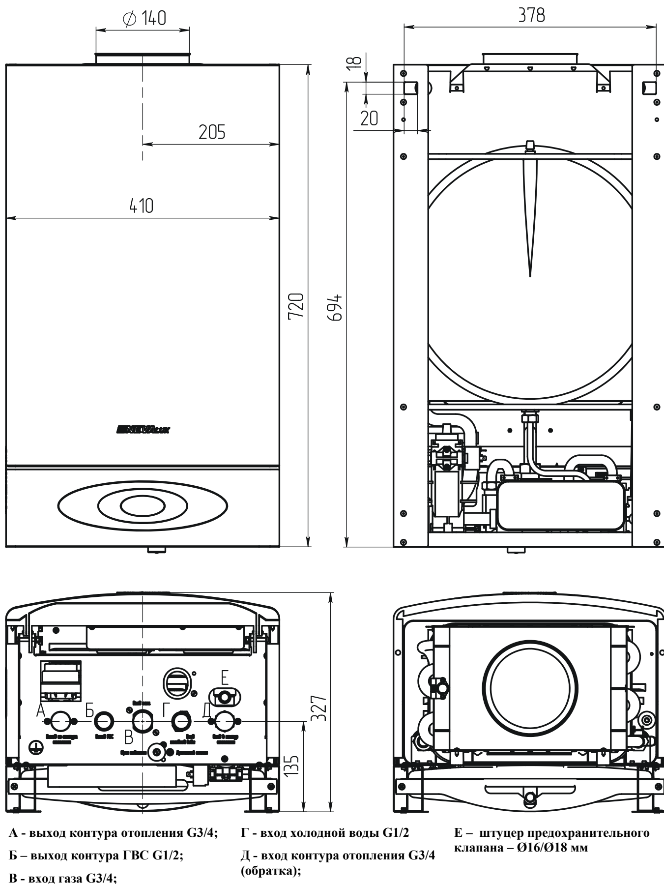
Рис. 1. Габаритные и присоединительные размеры котла
