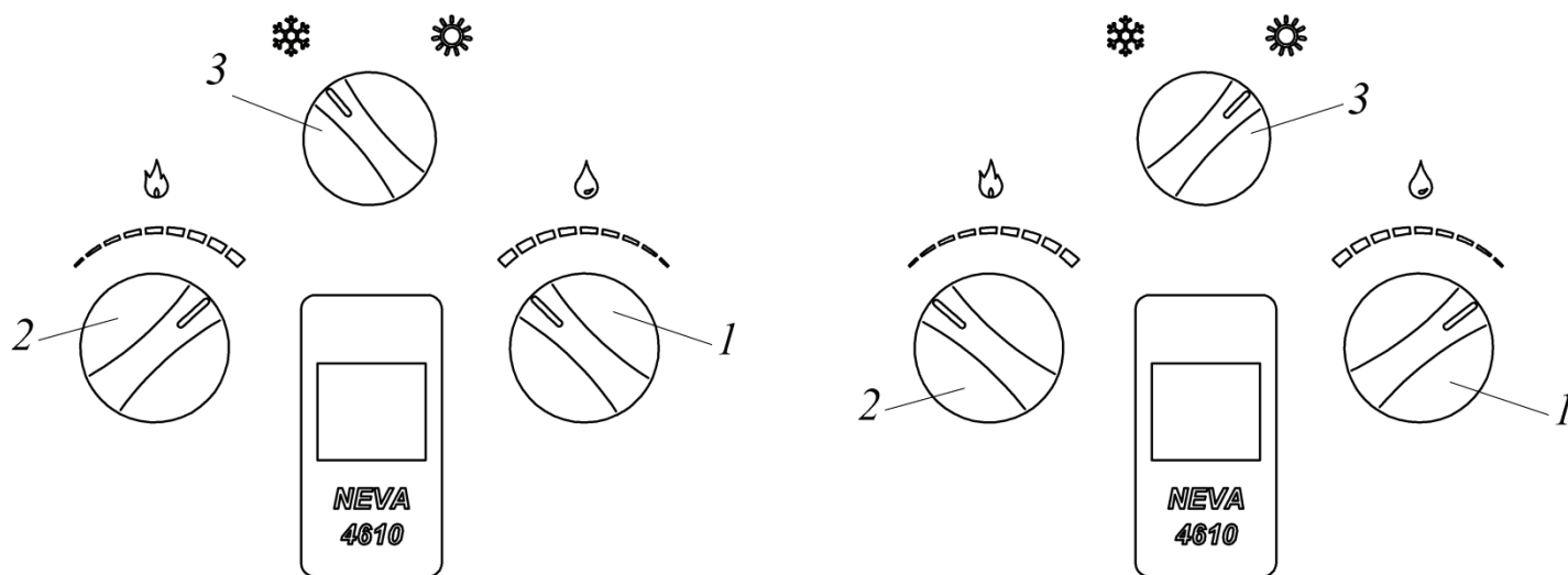
а) ручки регулировки расхода воды 1 и расхода газа 2 в положении «Максимальный расход» , ручка переключения режимов «зима-лето» 3 в положении «зима»
