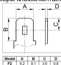
Размеры клемм/контактов F2
