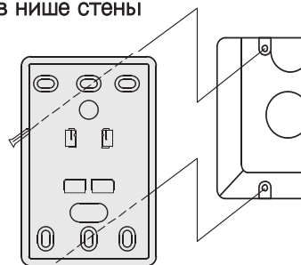
термостат кронштейн
