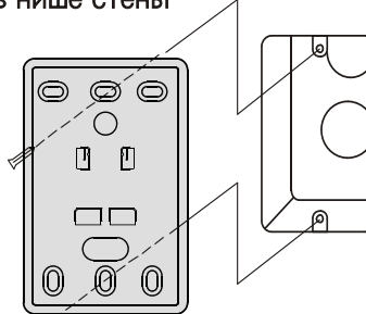
термостат кронштейн
