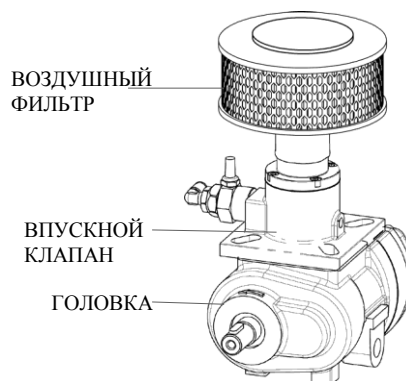
Рисунок 4.1: СИСТЕМА ВОЗДУХОЗАБОРА
