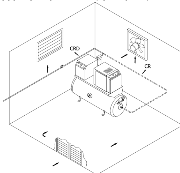
Рисунок 3.1: DMD С УСТАНОВКОЙ НА БАКЕ (CR & CRD), КОМПРЕССОРНАЯ И УСТАНОВКА
