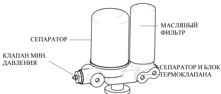
Рисунок 5.1: МАСЛЯНЫЙ ФИЛЬТР И СЕПАРАТОР
