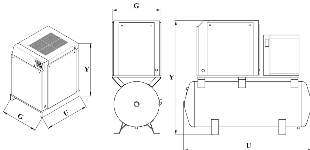
Рисунок 3.1: DMD SINGLE (C) & DMD НА БАКЕ (CR & CRD), РАЗМЕРЫ КОМПРЕССОРА
