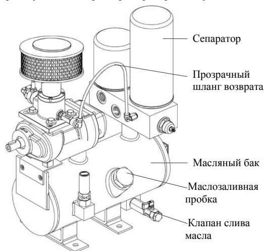
Рисунок 5.3: МАСЛЯНЫЙ БАК И ПАТРОН
