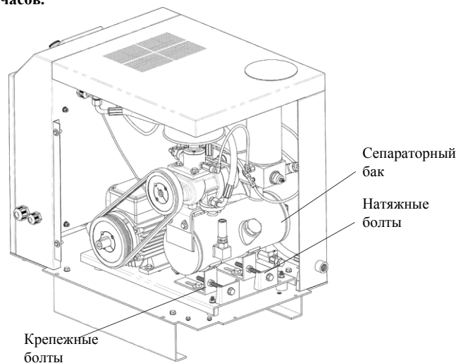
Рисунок 5.5: ЗАМЕНА РЕМНЯ И ТОЧКИ НАТЯЖЕНИЯ
