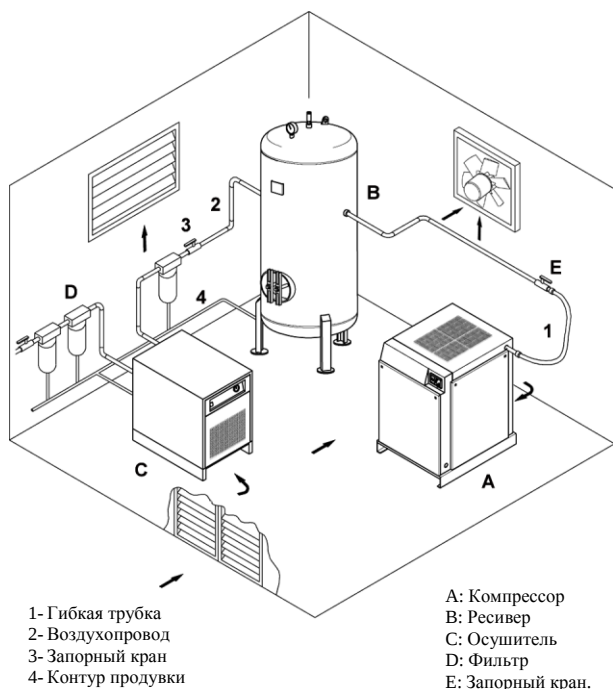
Рисунок 2.1: УСТАНОВКА
