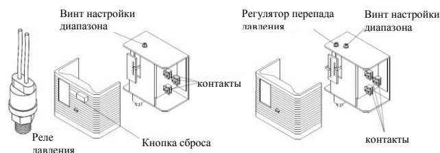
Рисунок 5.4: Регуляторы рабочего и защитного давления
