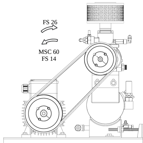
Рисунок 2.2: НАПРАВЛЕНИЕ ВРАЩЕНИЯ
