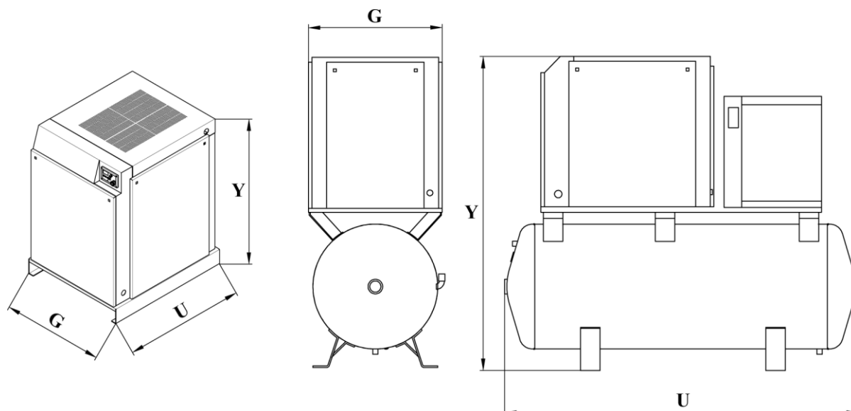
Рисунок 3.1: DMD SINGLE (C) & DMD НА БАКЕ (CR & CRD), РАЗМЕРЫ КОМПРЕССОРА
