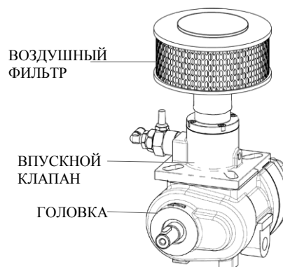
Рисунок 4.1: СИСТЕМА ВОЗДУХОЗАБОРА
