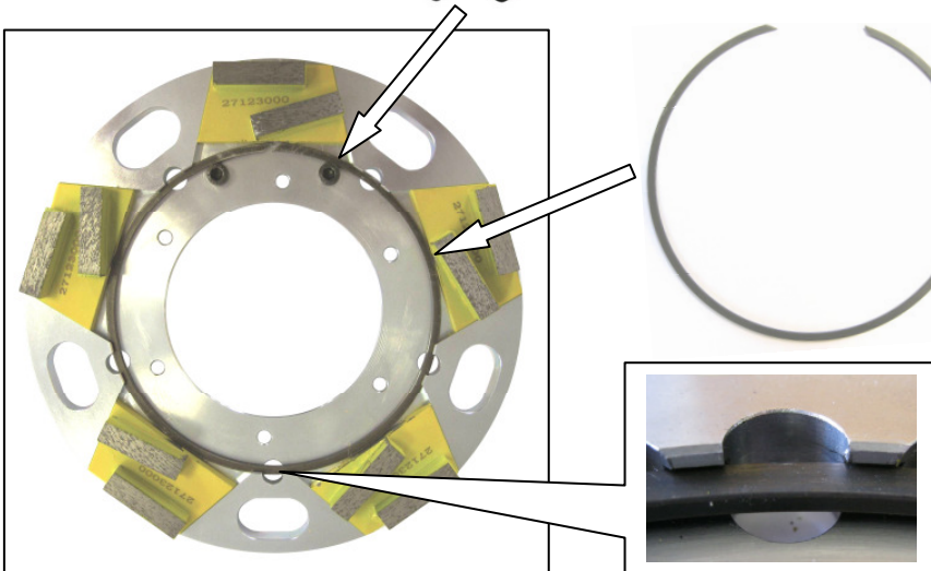
2 Sicherungsschrauben M6x6
