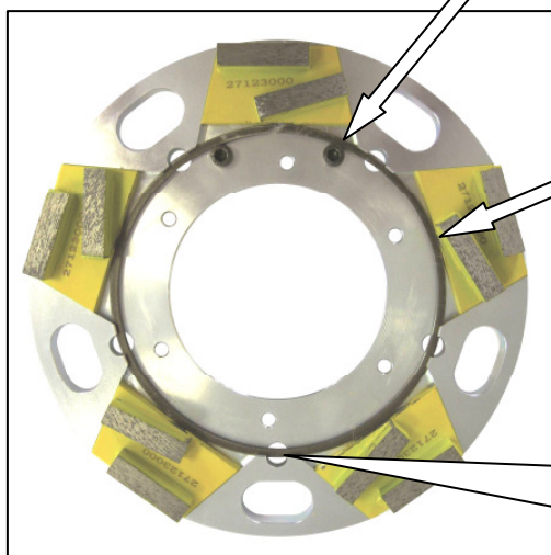
2 borgschroeven M6x6
