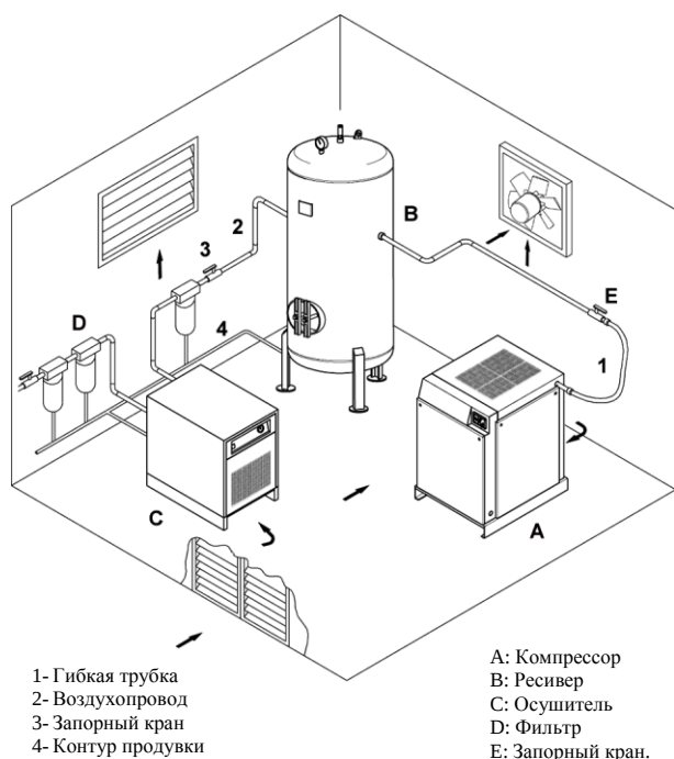
Рисунок 2.1: УСТАНОВКА
