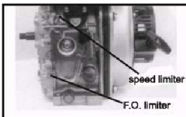
Ограничитель оборотов
