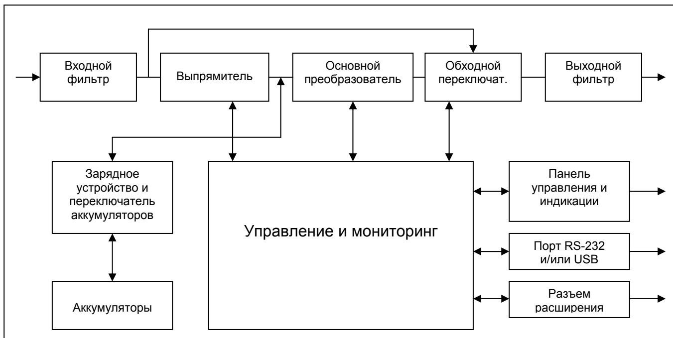
рис. 1. Блок-схема ИБП
