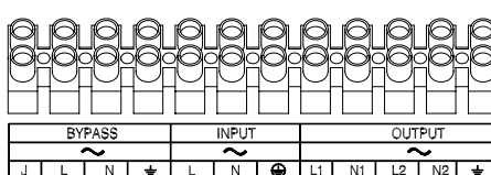
VGД 4/5/6K-ISO TB
