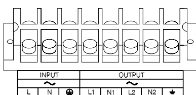
VGД 4/5/6/8/10/12K-ISO TB
