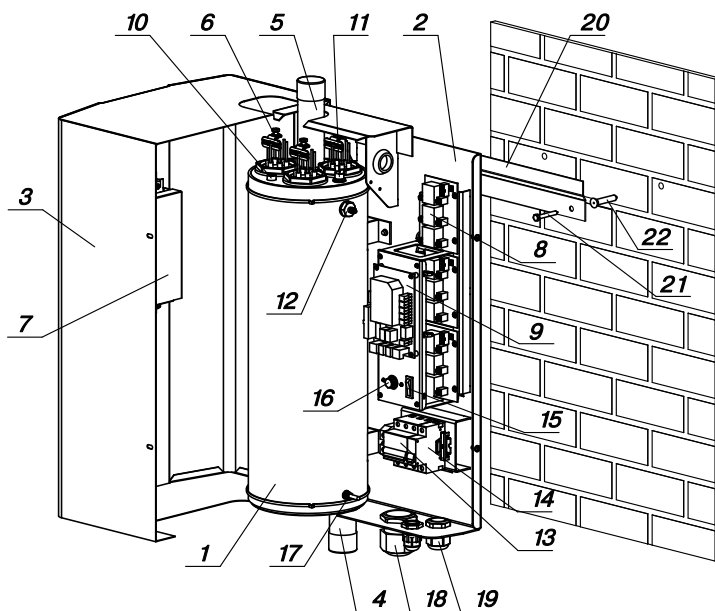
Рис. 1. Конструкция водонагревателя и способ его крепления к стене
