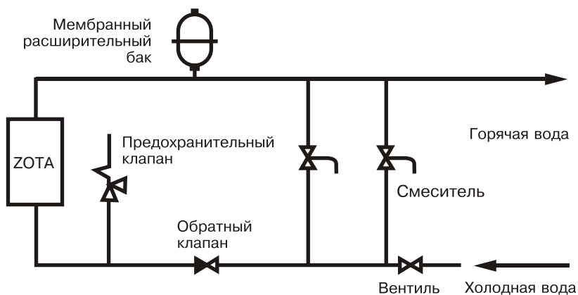
Рис.5 Упрощенная схема подключения в качестве водонагревателя с проточным режимом работы
