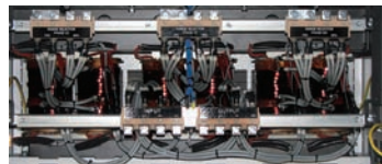
Вольтодобавочные трансформаторы
