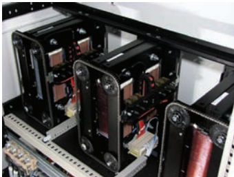
Регулируемые автотрансформаторы (регуляторы напряжения) с двухсторонними дифференциальными токосъемниками на цепной передаче (высокоскоростные, высоконадежные)
