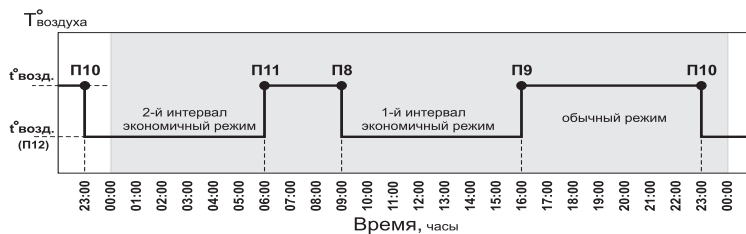
Рис.4 График температуры воздуха в помещении для Режим 1.
