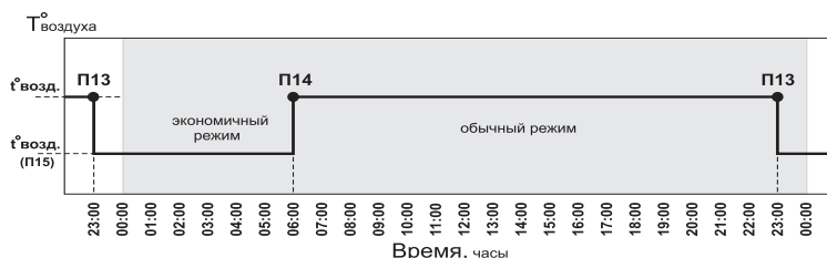
Рис.5 График температуры воздуха в помещении для Режим 2.
