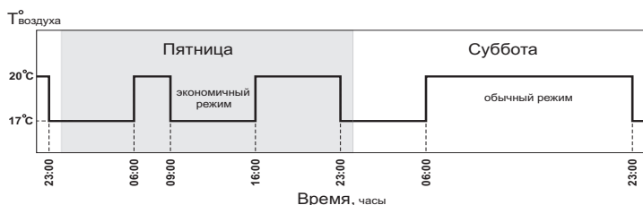
Рис.6 График температуры воздуха в помещении для Режим 3.
