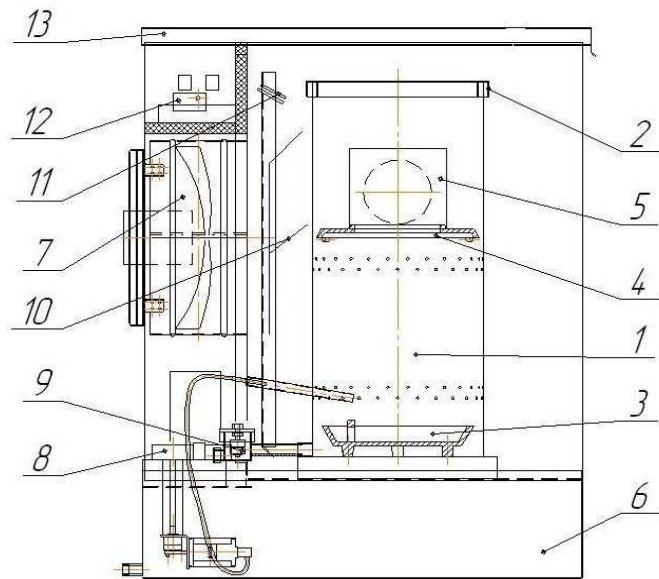
Рис.3 Схема отопителя
