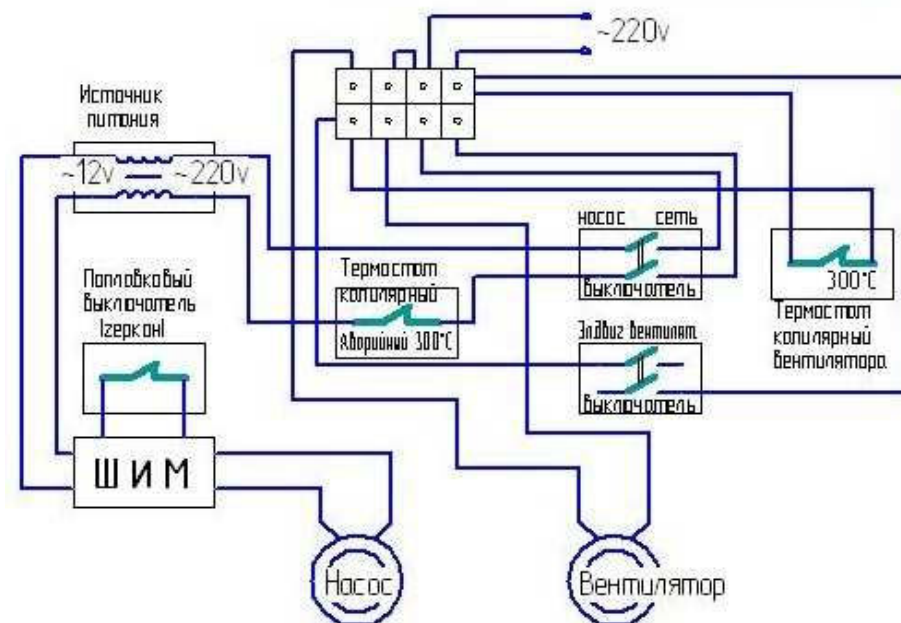
Рис.2 Схема отопителя электрическая
