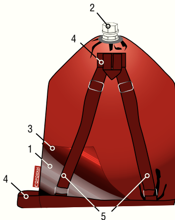
Рисунок 2 – Устройство канистры
