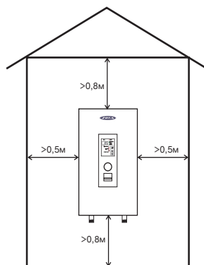
Рис.4 Схема установки миникотельной
