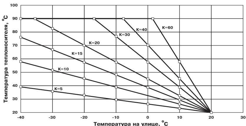
Рис.7 График погодозависимого регулирования.
