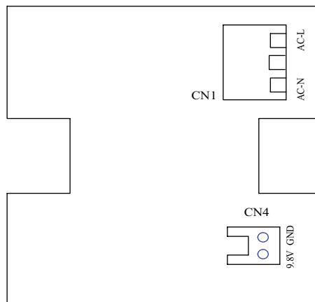
Рис. 6.22 Подключение электропитания
