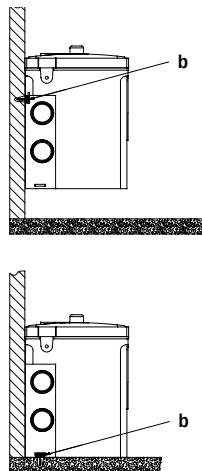
Установка насосного устройства на стене и на полу
