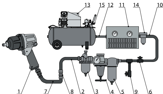
Рисунок 3. Подключение пневматики.
