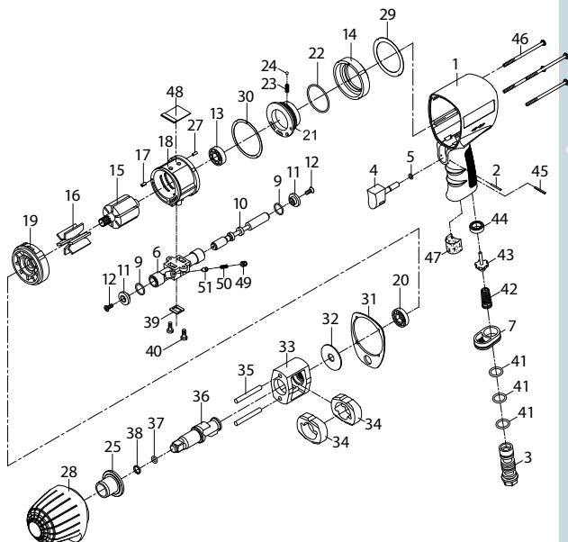
Рисунок 2. Деталировка.
