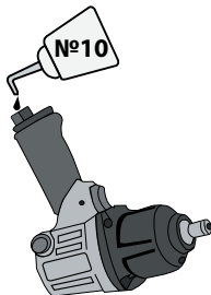
Рисунок 4. Смазка инструмента.
