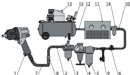
Рисунок 3. Подключение пневматики.
