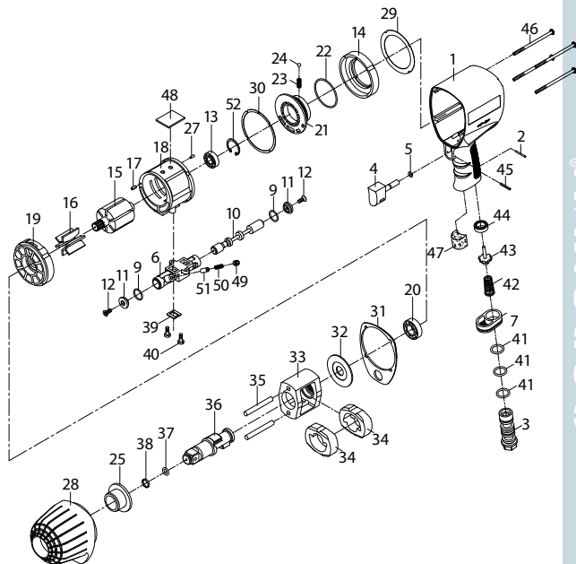
Рисунок 2. Деталировка.
