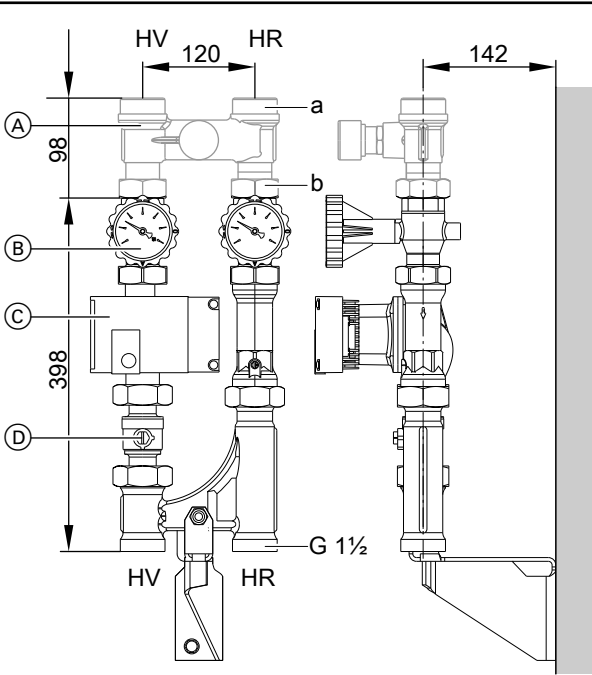
Регулятор отопительного контура Divicon без смесителя (настенный монтаж, изображение без теплоизоляции)
