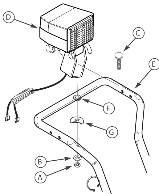
Сборка фары
