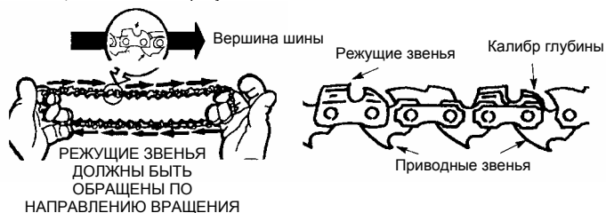
Установка шины
