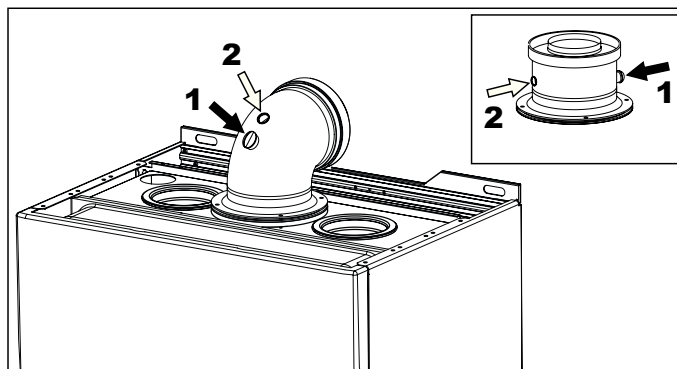
рис. 30 - Анализ дымовых газов
