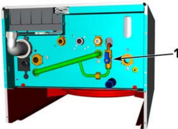
рис. 15 - Кран для заполнения системы отопления
