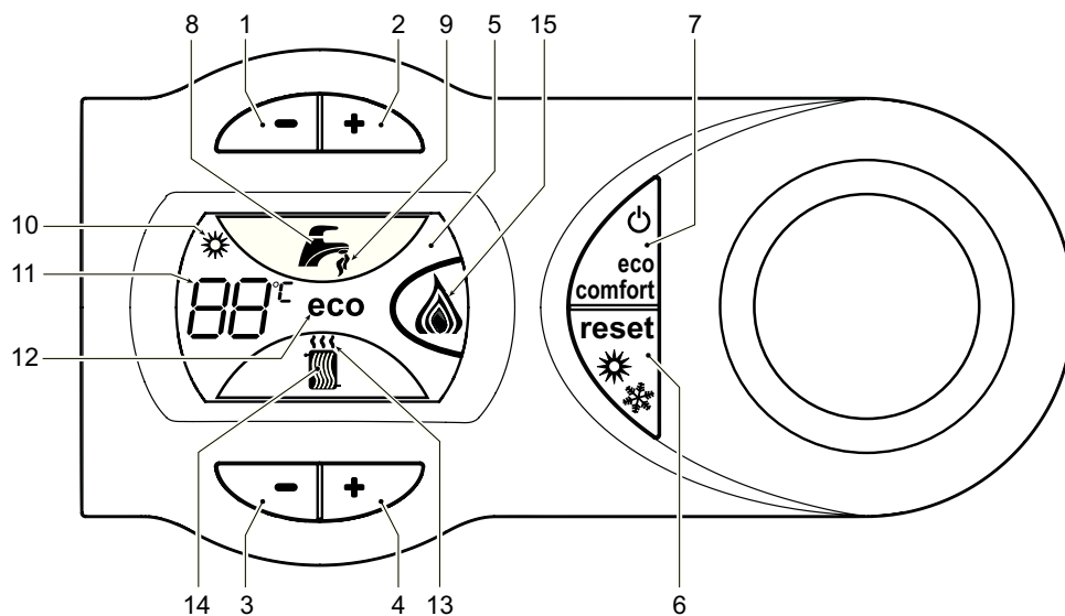
рис. 1 - Панель управления
