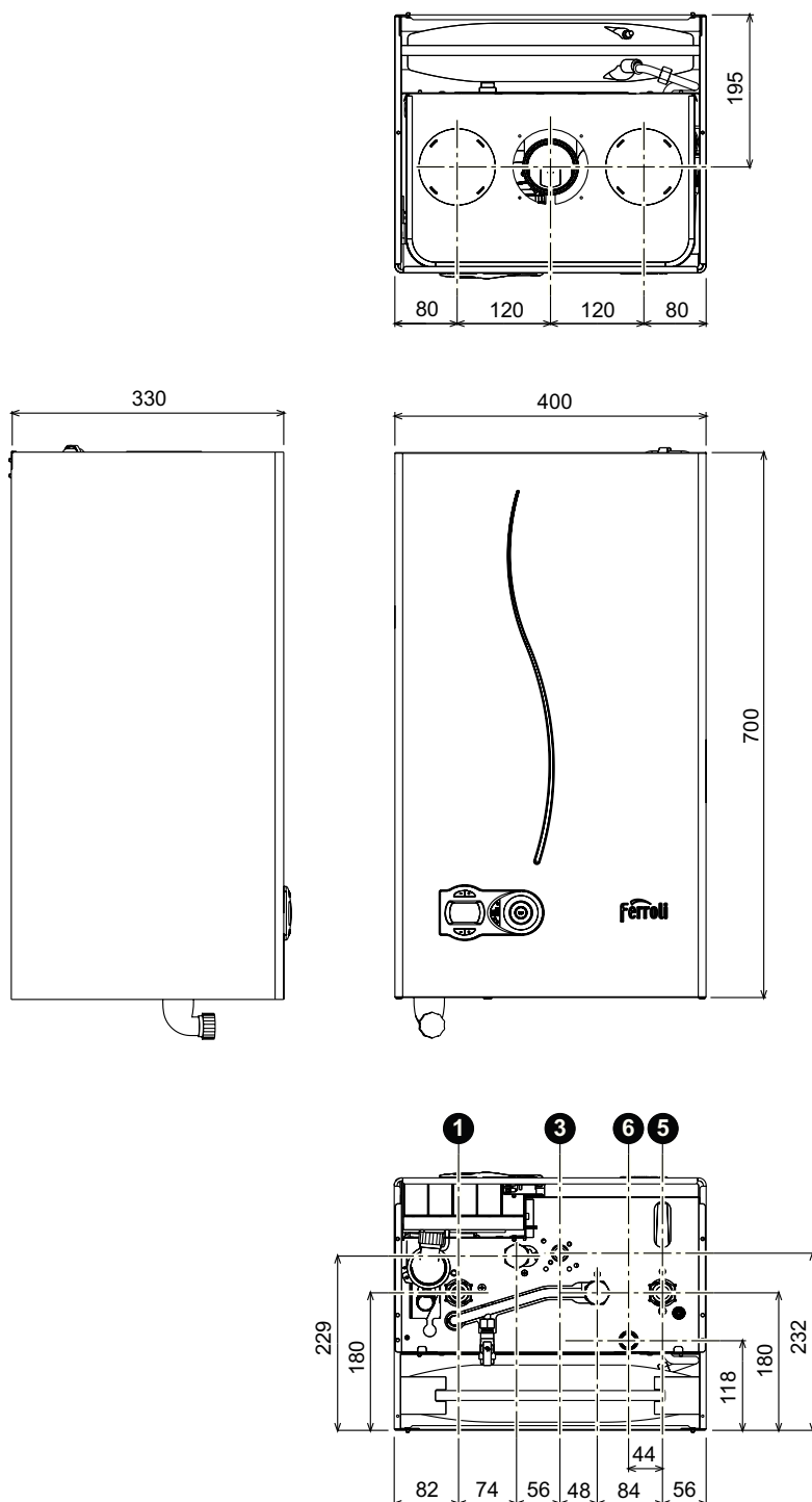
рис. 31 - Габаритные размеры и присоединения
