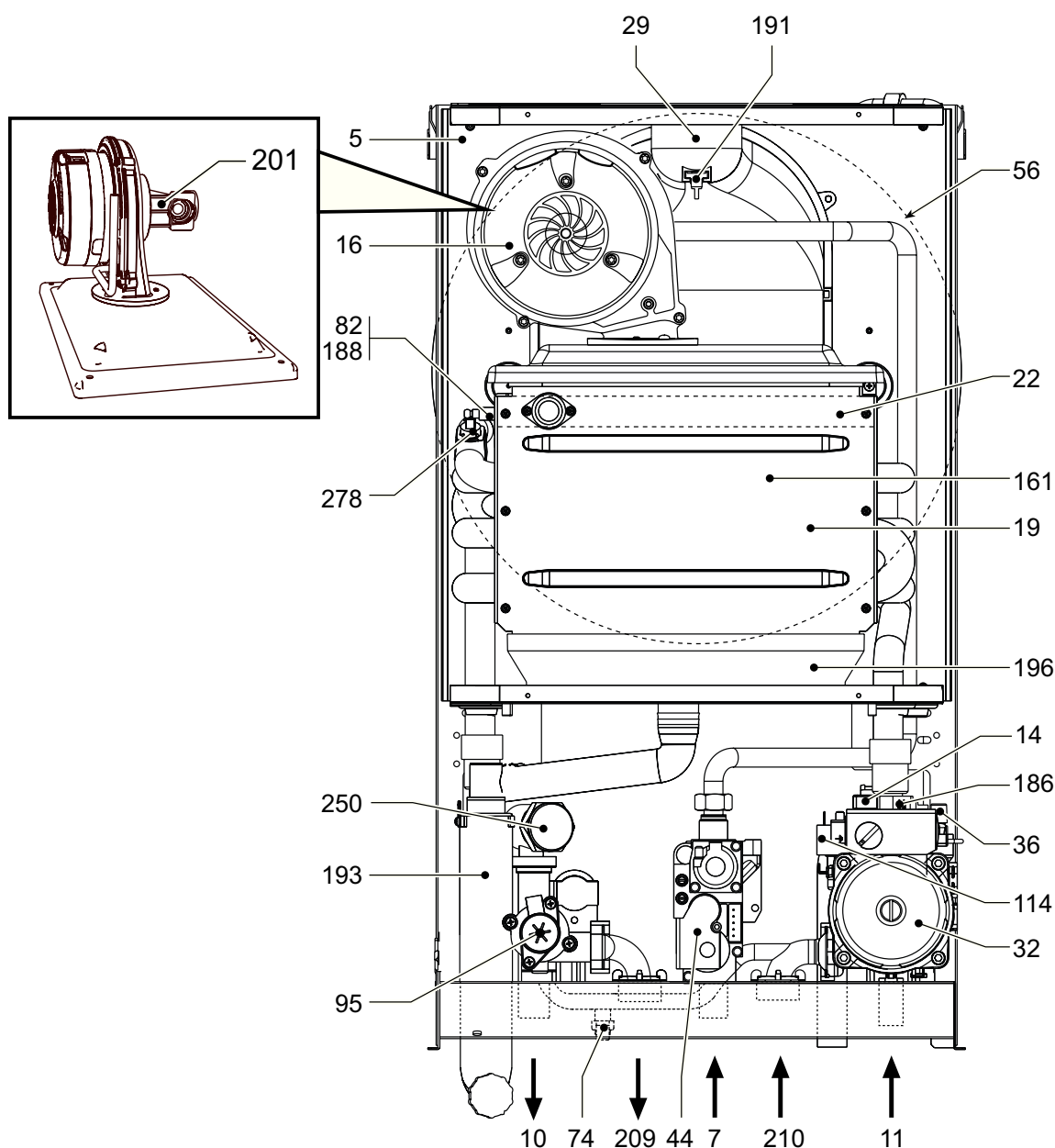
рис. 32 - Общий вид
