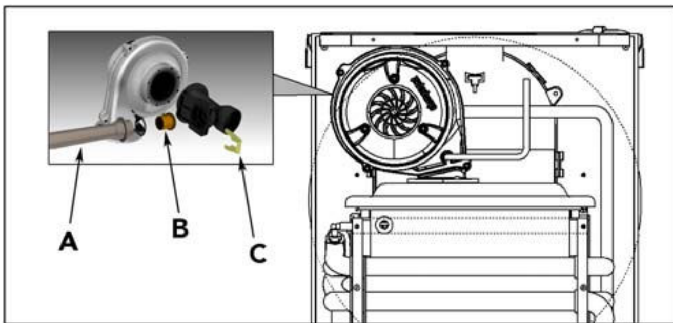
рис. 27 - Перенастройка котла на другой вид газа
