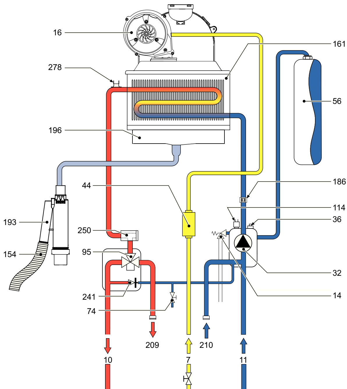
рис. 33 - Схема системы отопления и ГВС
