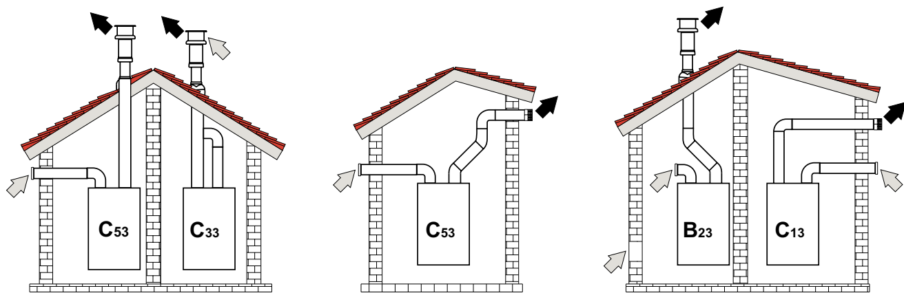
рис. 23 - Примеры присоединения с помощью отдельных труб (⇐ = Воздух / ➡ = Дымовые газы)
