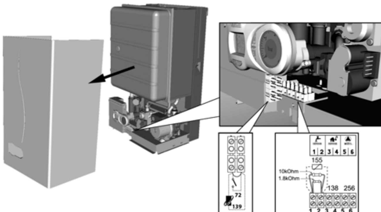
рис. 19 - Доступ к блоку зажимов
