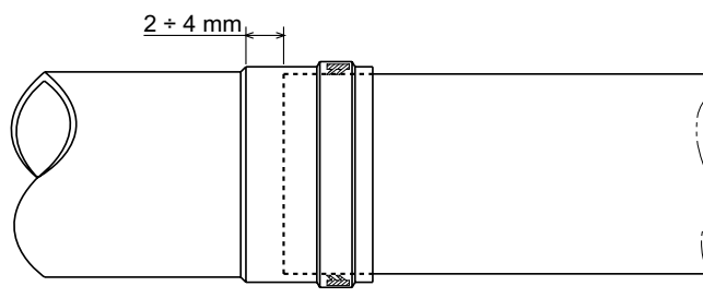
рис. 20 - Тепловое расширение
