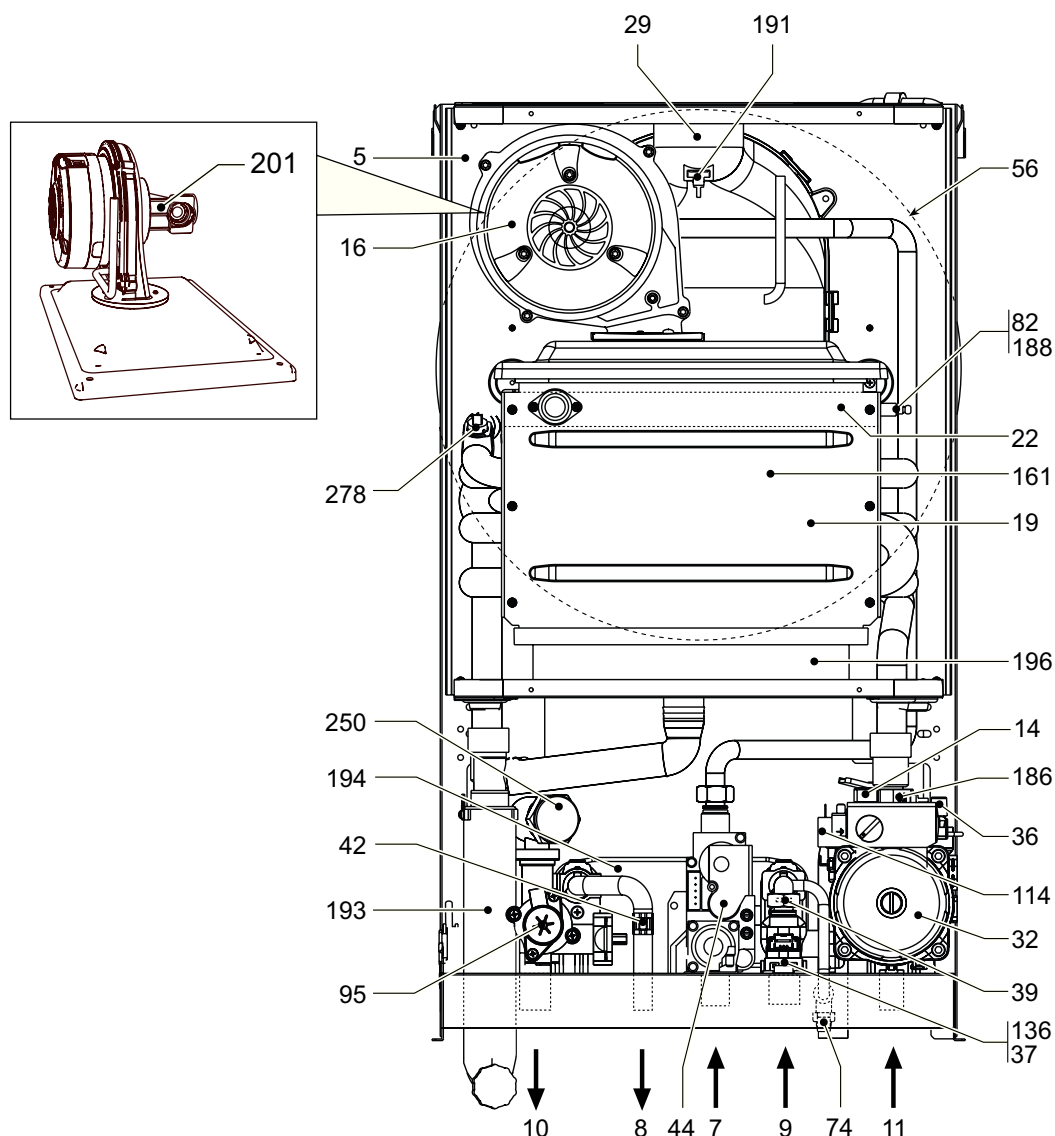
рис. 31 - Общий вид
