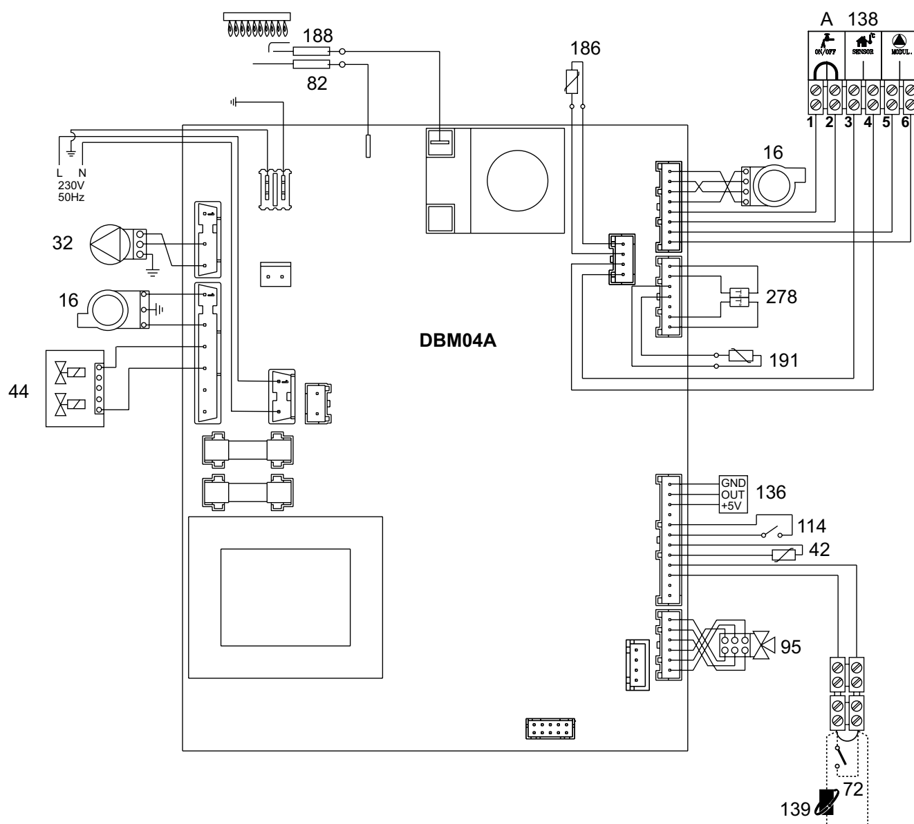
рис. 33 - Электрическая схема
