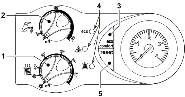
рис. 1 - Панель управления
