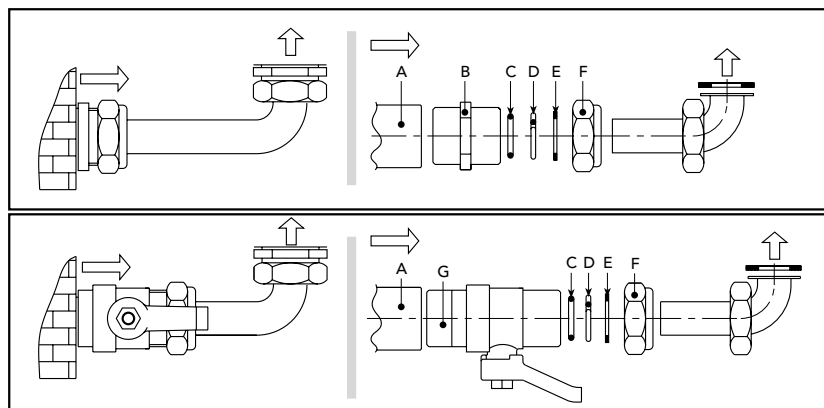
рис. 7 - Соединительный комплект
