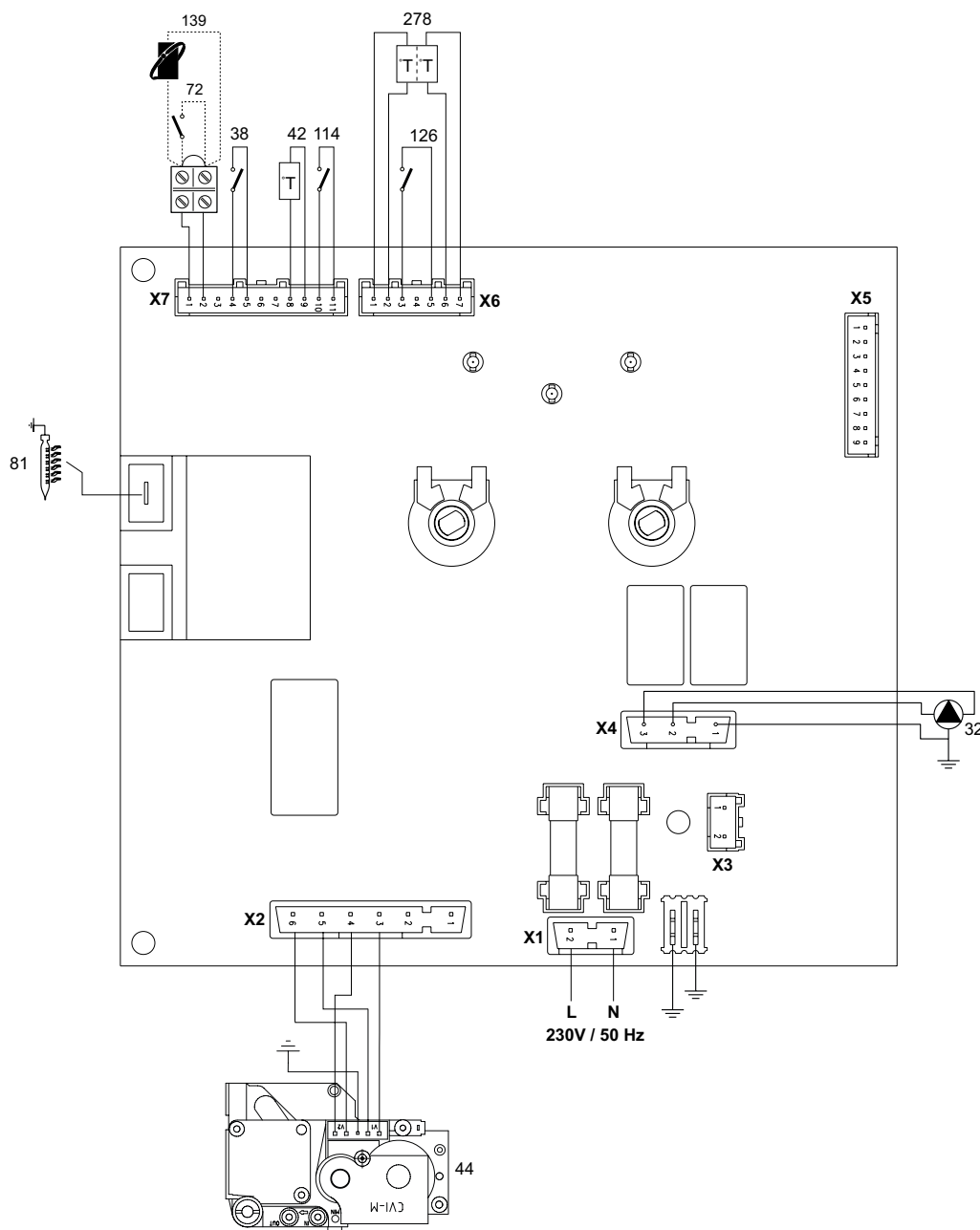
рис. 15 - Электрическая схема
