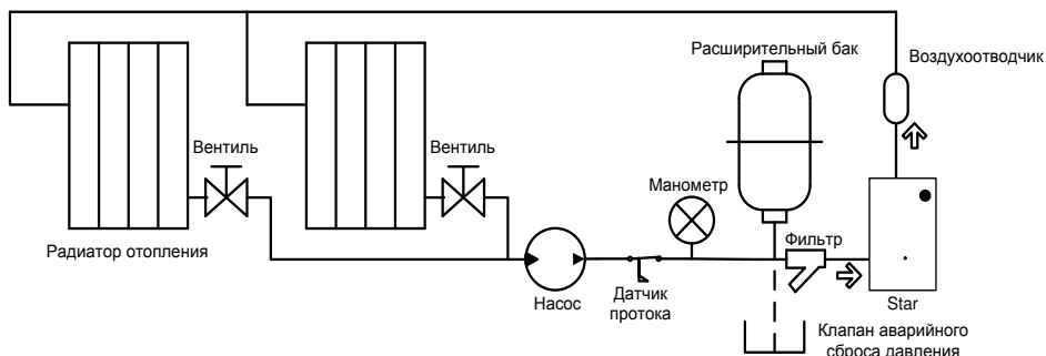
Рнс.4 Обнщнй внд снстемн отопленнн с прннуднтельной цнркуляцней теплоноснтеля.
