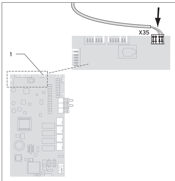
1 Гнездо X35
