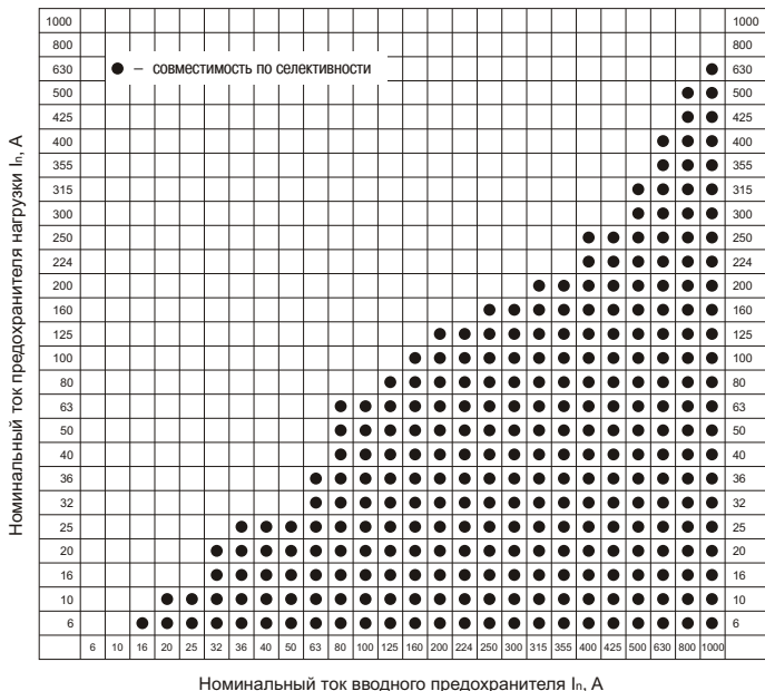
Рисунок 5 Номинальные токи предохранителей для совместного межуровневого использования
