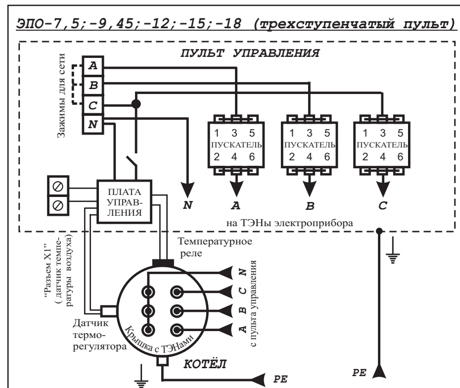
Рисунок 8 - Электрическая схема подключения
