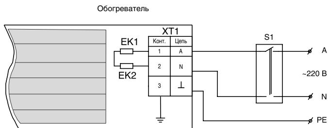
Рис. 2. Обогреватель ВИН-2.0
