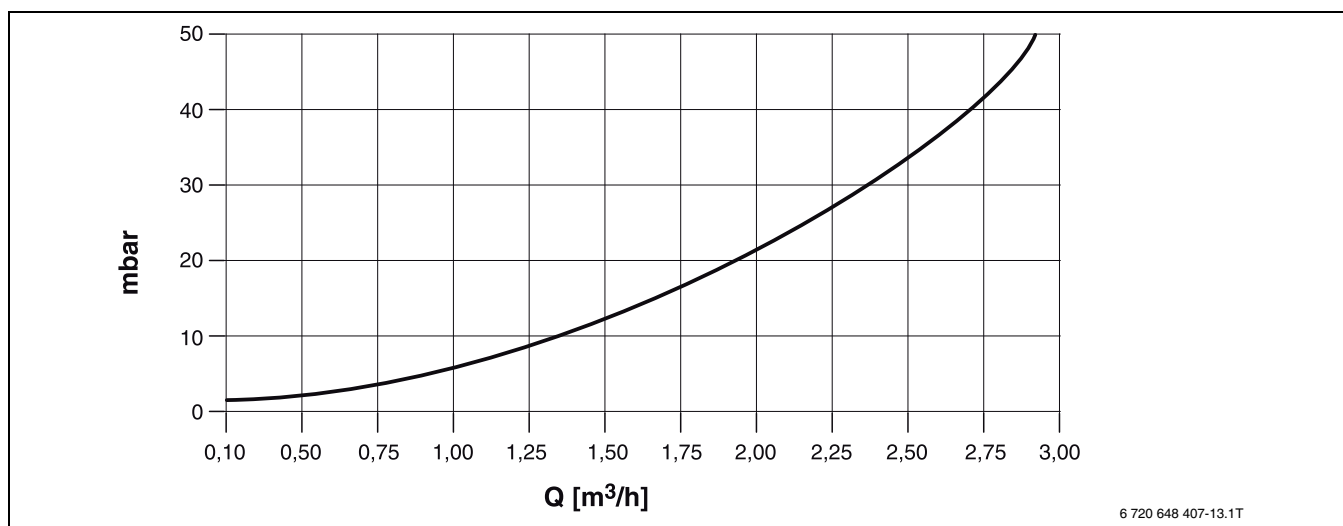
Рис. 5 Гидравлические потери давления (мбар) в зависимости от объёмного расхода ( \text{m}^3/\text{ч} )
