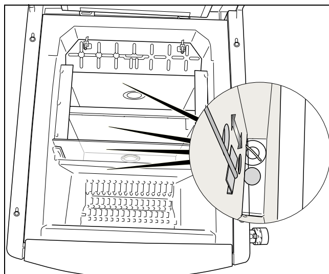
Рис. 23 Чистка стенок
