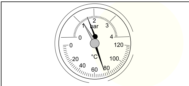
Рис. 36 Термоманометр
