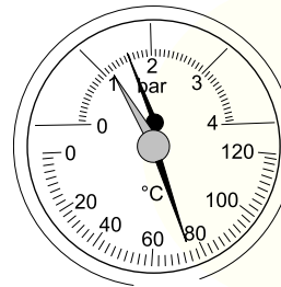
Рис. 25 Термоманометр
