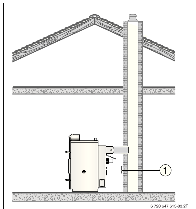
Рис 16 Расположение регулятора подачи дополнительного воздуха
